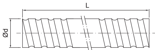
図 2.3.1 ねじ見取り図
