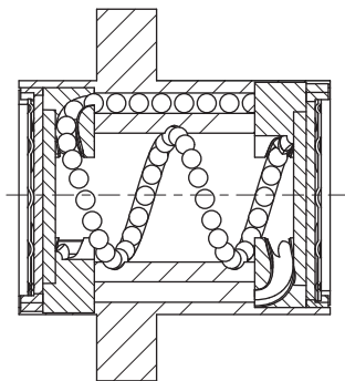
図 1.6.4 Y, YA, H, A タイプナット
